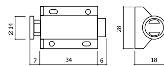
FECHO MAGNÉTICO MAGNETIC BOLT
