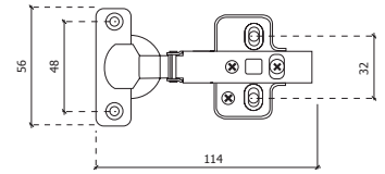
C/AMORTECEDOR W/DAMPER
